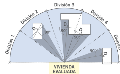
↑ Figura 6.11 Medición de distancia D para determinación del FAR
