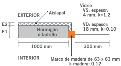
↑ Figura 6.3 puente térmico P05 asociado a ventanas
