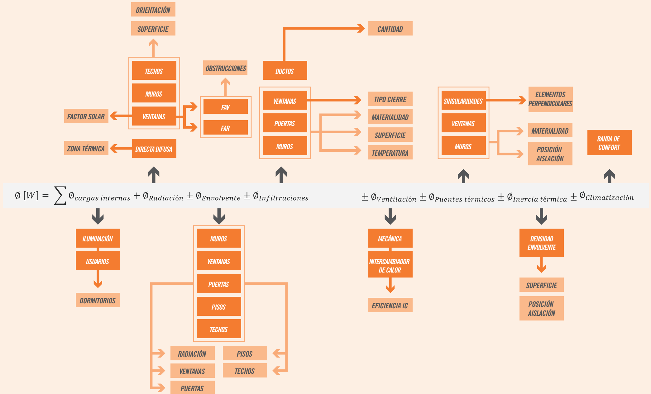
↑ Figura 18.4 Diagrama de variables y subvariables asociadas al flujo térmico
