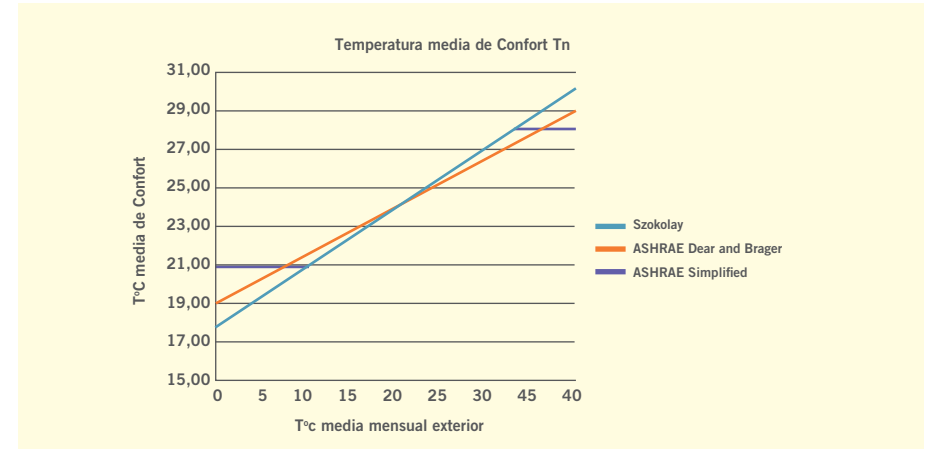
↑ Figura 18.20 Temperatura de confort neutral T n .
