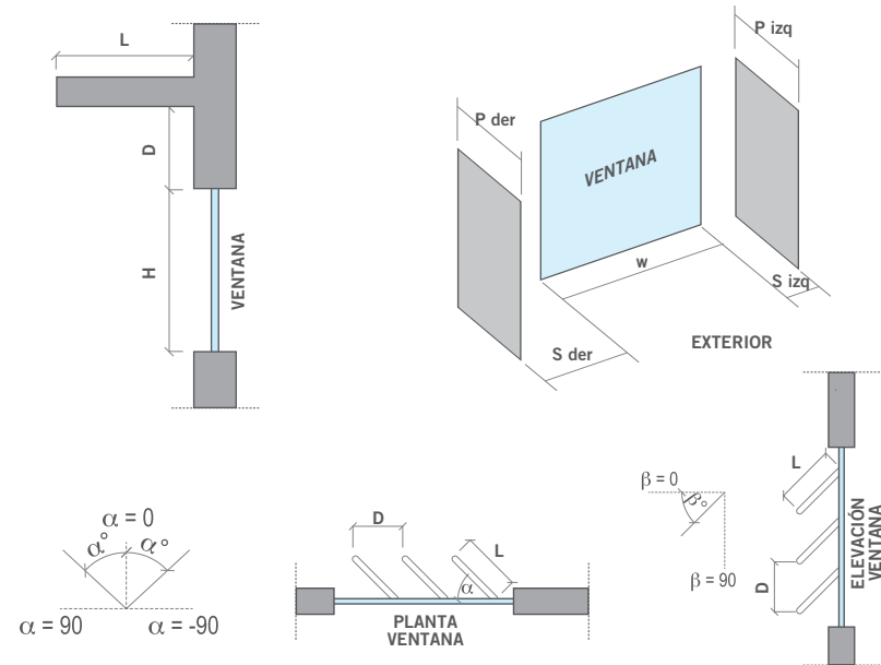
↑ Figura 18.7 Tipologías de obstrucciones particulares de cada ventana
