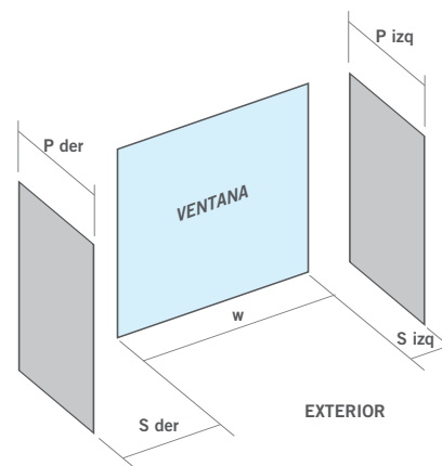
↑ Figura 6.7 Ejemplo de FAV 2
