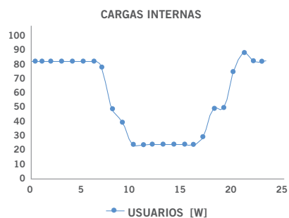
Figura 7.2 Cargas internas por usuarios
