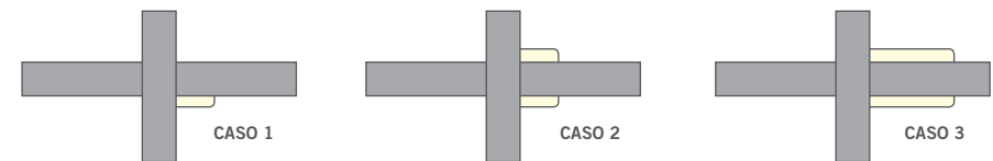
↑ Figura 18.17 Esquemas de los tres casos a aislación considerados para el puente PO4. La banda amarilla corresponde a una capa de aislante. En todos los casos se supone que el aislante está por el lado externo, es decir en la proyección hacia el exterior.
