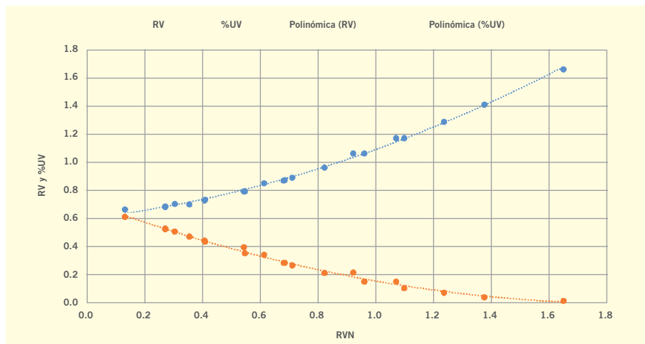
↑ Figura 18.13 Relación entre RV, %UV y RVN a usar en la calificación.
