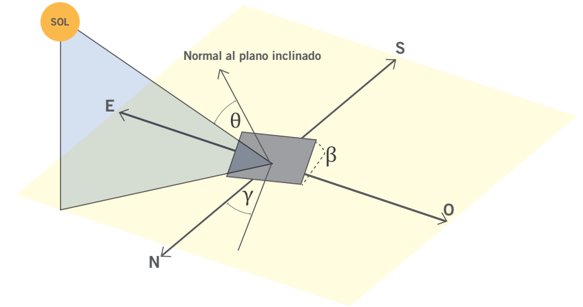
↑ Figura 18.6 Ángulos definidos para la definición de un plano inclinado con respecto a un plano horizontal.
