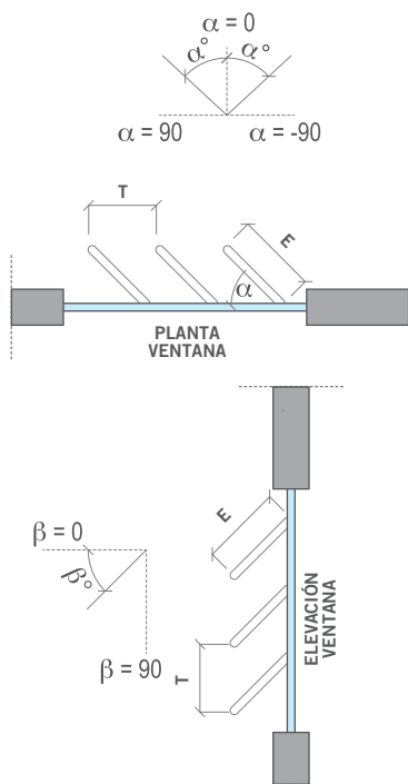
↑ Figura 6.8 Ejemplo FAVs 3
