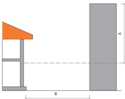
↑ Figura 6.12 Corte ejemplo para medición del parámetro A [m]
