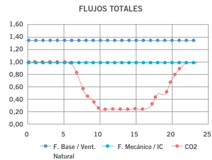
↑ Figura 7.3 Flujos de aire mínimos
