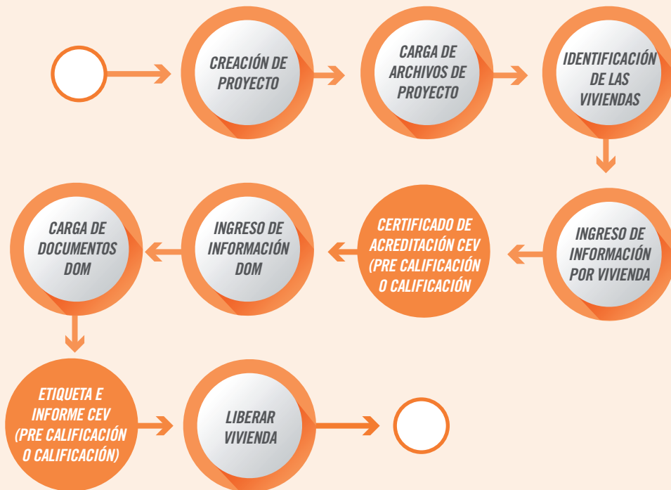
↑ Figura 13.1 Flujo de sistema web CEV
