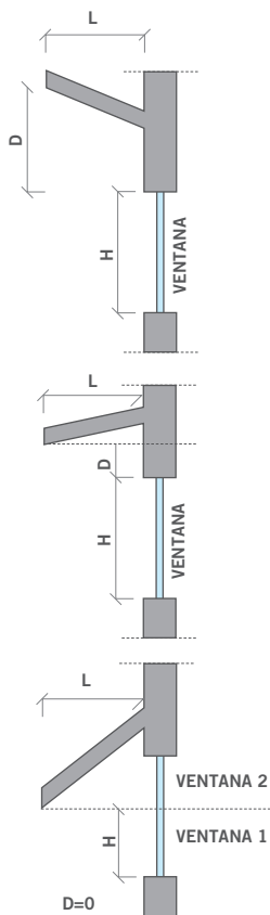
↑ Figura 6.6 Distintas elevaciones de aleros FAV 1
